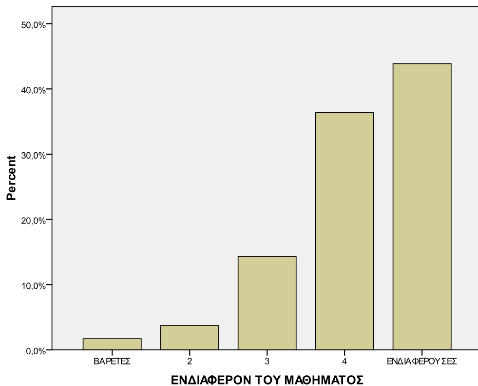
Σχήμα 30. Ενδιαφέρον μάθημα.
